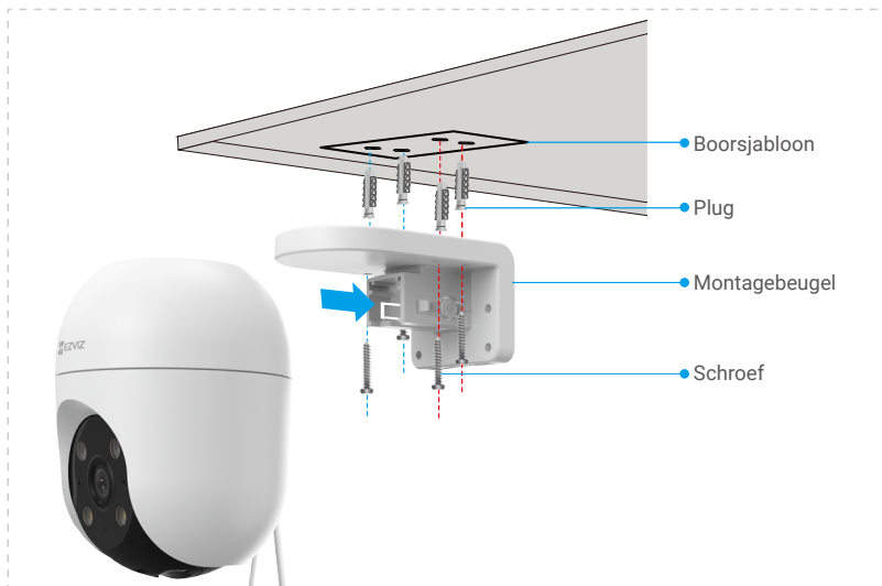
Afb. 1 Plafondmontage
