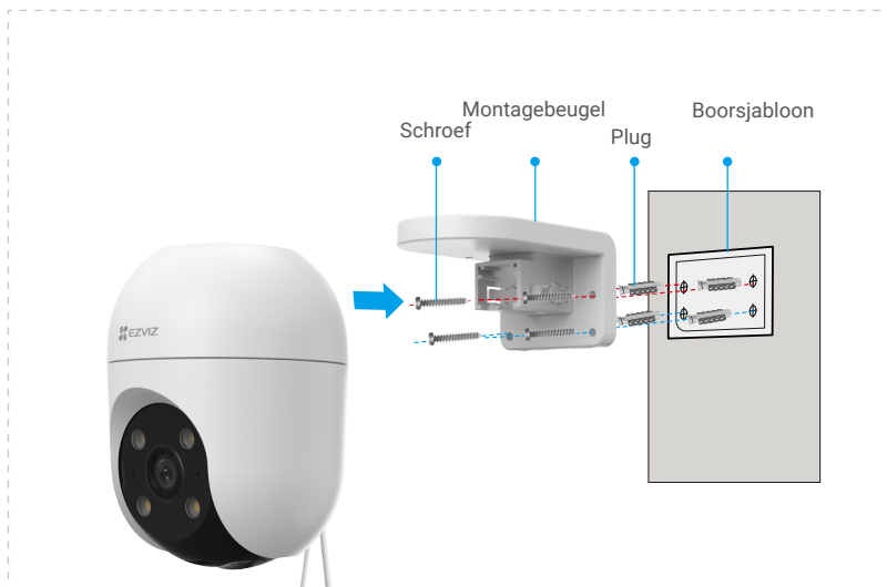
Afb. 2 Muurmontage
